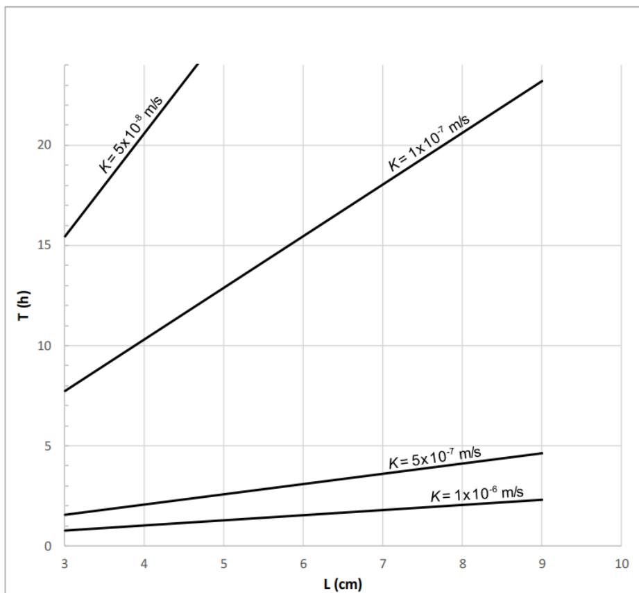
Figur 5. Diagram för avläsning av hydraulisk konduktivitet från perkolationsstest när sjunktiden är i tidsspännet timmar. Observera att diagrammet endast är giltigt om testet är utformat så att H_0/H_1 \approx 1,2 .
