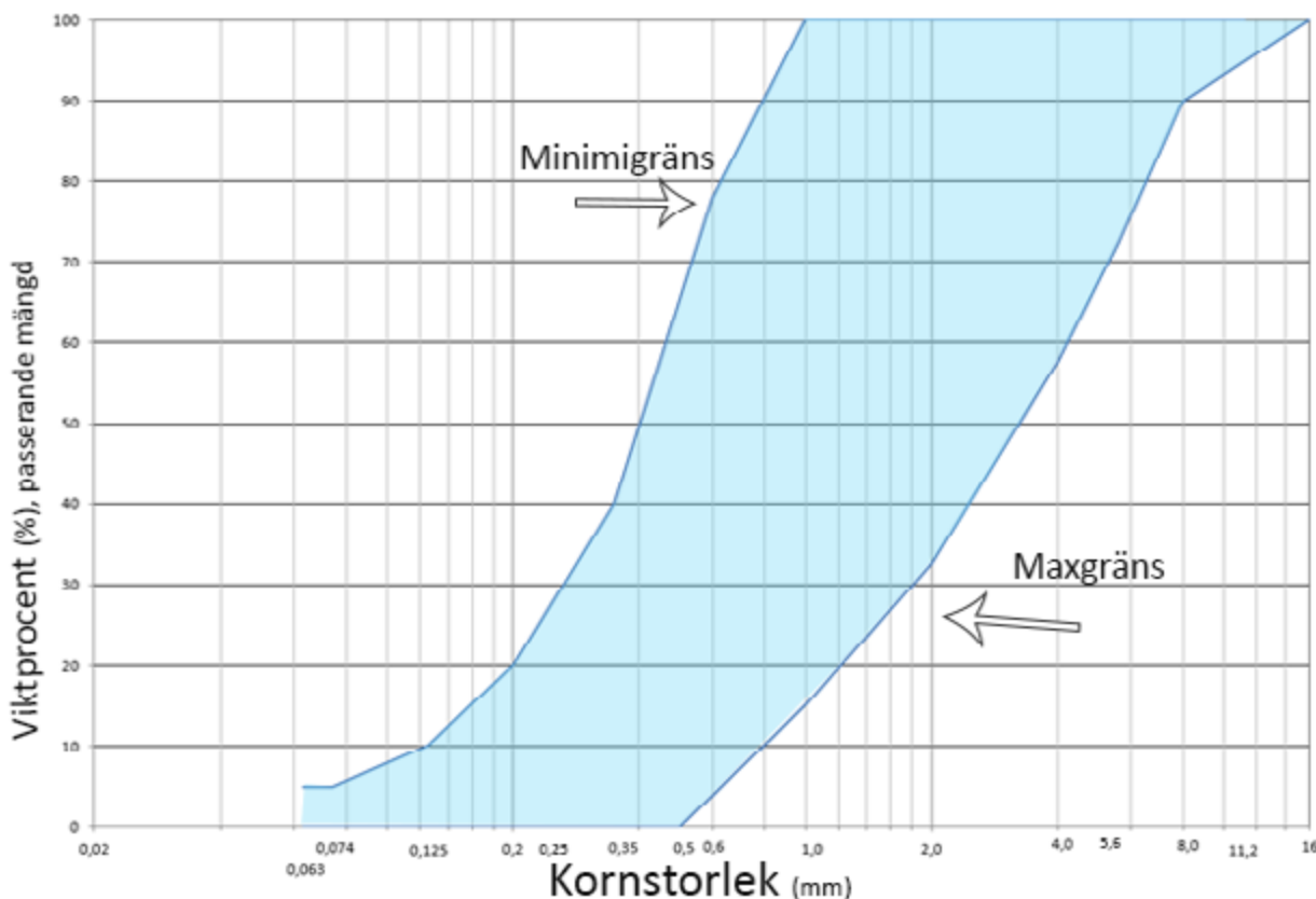
Figur 1 Rekommenderade gränser för blandning av kornstorlekar i markbäddssand som filtermaterial i markbäddar och som förstärkningsmaterial vid infiltration.
