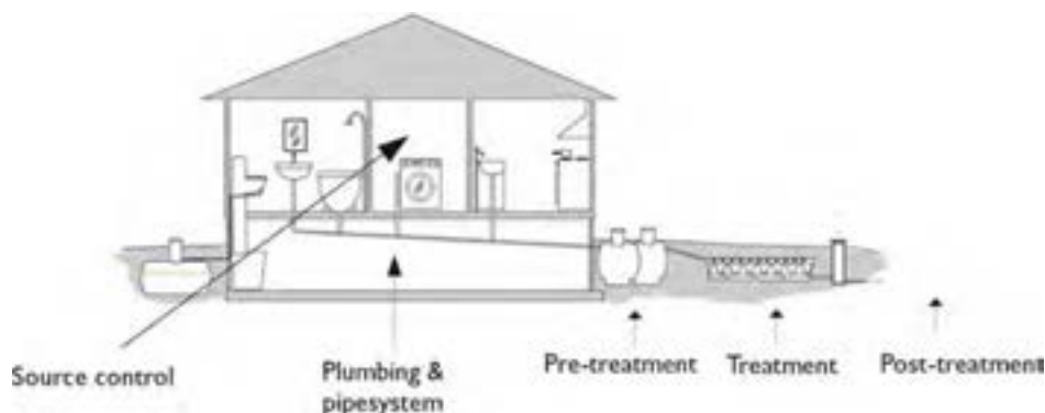
Figur 6. Ett avloppssystem kan uppdelas i fem delkomponenter, nämligen källorna, ledningssystemet, förbehandlingen, behandlingen och bortledningen. Bilden visar ett källsorterande system med behandling av BDT-vatten i en innesluten markbädd (Ridderstolpe, 2004).
