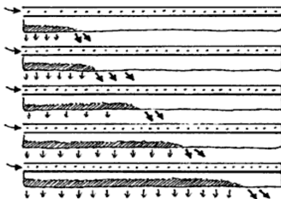
Figur 8. Principen för så kallad progressive clogging innebär att vatten sprids över filterytan och skapar goda förutsättningar för omättad strömning (Khan et al. 2007).
