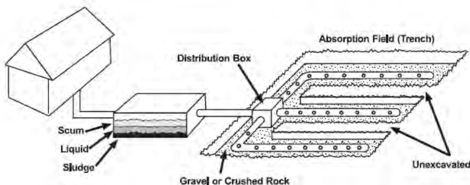
Figur 4. Den amerikanska modellen för markbaserad rening inkluderar en slamavskiljning som tillåter långtidslagring och mineralisering av slam samt infiltration i mark där vattnet fördelas genom i smala diken (USEPA 2003).
