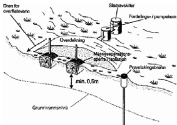
Figur 3. I Norge är infiltration en av de vanligaste typerna av rening för enskilda avlopp. Vanligt är att dessa bäddar är byggda som smala och ytligt förlagda diken till vilket slamavskiltat vatten pumpas. Norska dimensioneringsgrunder innebär också att anläggningar normalt belastas med lägre vattengivor än i Sverige.
